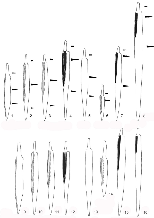
Рис. 2. Типы и варианты ножей-кинжалов по Я. Прасолову: 1 – тип 0, 2 – тип 1а, 3 – тип 1б, 4 – тип 2б, 5 – тип 2а, 6 – тип 2б, 7 – тип 3а, 8 – тип 3б, 9 – тип 0 (так наз. (боевой) нож с горбатой спинкой), 10 – тип 1, вар. А, 11 – тип 1, вар. б, 12 – тип 2, «классический» нож-кинжал, 13 – тип 2, вар. А, 14 – тип 2, вар. б, 15 – тип 3, вар. а, 16 – тип 3, вар. б (Prassolov 2018: Abb. 33, 34)
